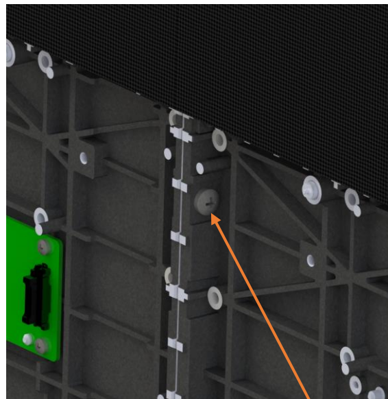
M5 X 10 PHMS
